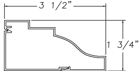
Base M1984 Trim M20548
