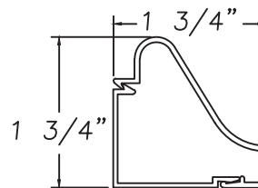
Base M15266 Trim M19136
