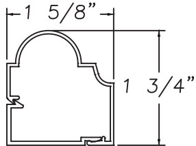
Base M2144 Trim M20526
