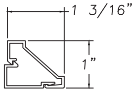
Base M20546 Trim M20545
